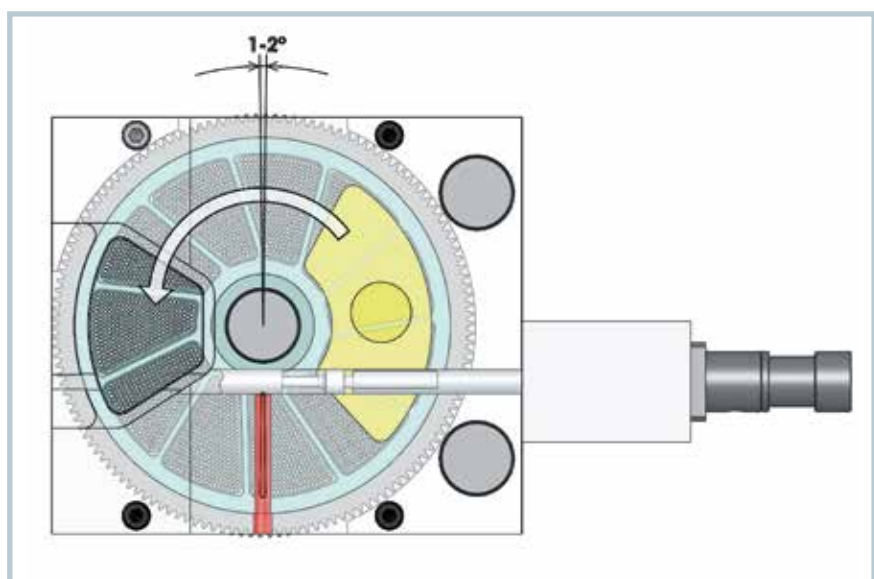
Bild 9. Technischer Aufbau des Rotary-Filterationssystem RSFgenius (Bild: Gneuß)
